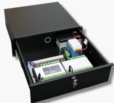
19"-Schublade, geöffnet
