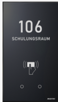
Zutrittsleser mit schwarzer Glasplatte (RAL 9005), Zimmernummer, Zimmerbezeichnung, DND, MUR, ohne Klingel
